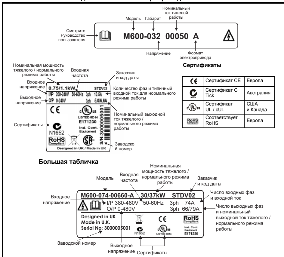
Рис. 2-2 Типичные заводские таблички электропривода
